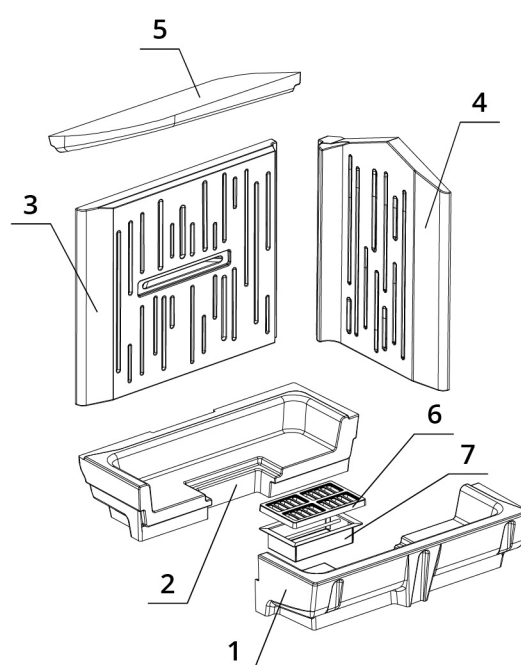
Carcon Feuerraum
